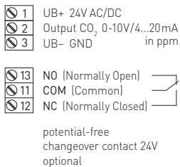
Схема подключения
